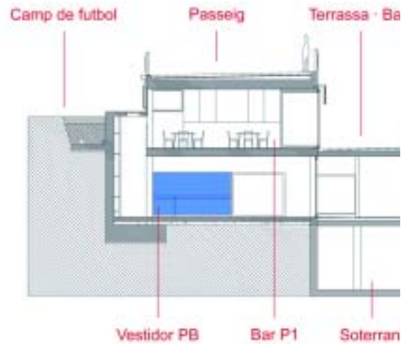
Mapa de secció de la Nova Piscina Municipal del Papiol
